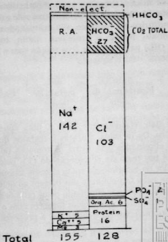
FIG. 1 — (Modificado de Bland, J. H. 2 ) — Diagrama da estrutura eletrolítica do plasma, mostrando na coluna da direita os cátions e na da esquerda, os ânions. Na coluna de cátions, o traço interrompido limita a reserva alcalina (R. A.). Isto é, a quantidade de base disponível para neutralizar o bicarbonato do plasma (em achurado — 27 mEq/litro). O CO 2 libertado pelo bicarbonato e pelo ácido carbônico corresponde ao CO 2 total.
